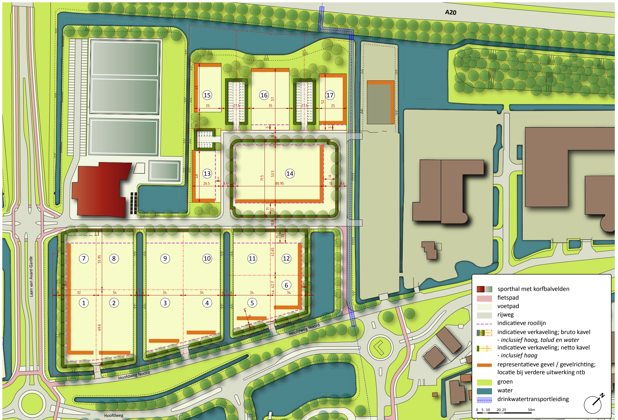
stedebouwkundig plan bedrijvenpark “Kleine Vink”; plankaart
