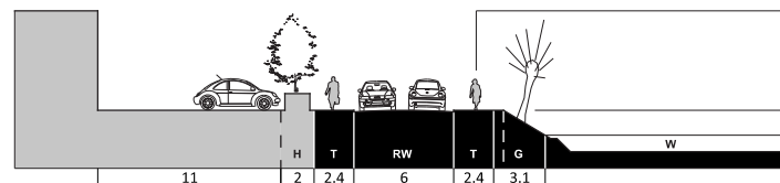
PROFIEL A - A
