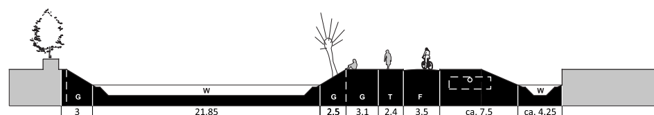
PROFIEL C - C
