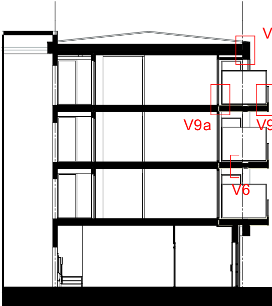
Doorsnede B
