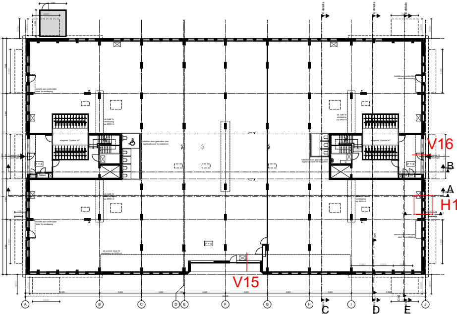
Begane grond
