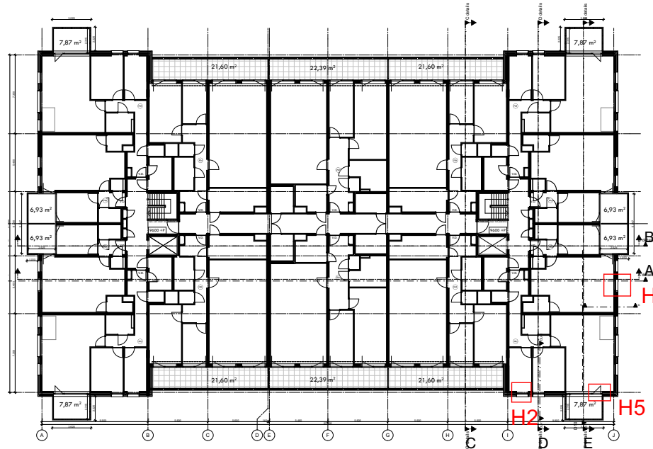
3e verdieping
