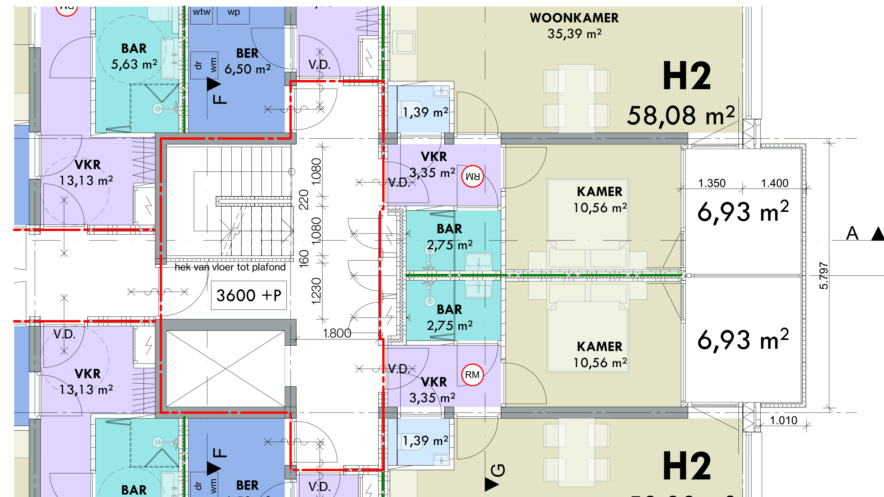
1e verdieping
