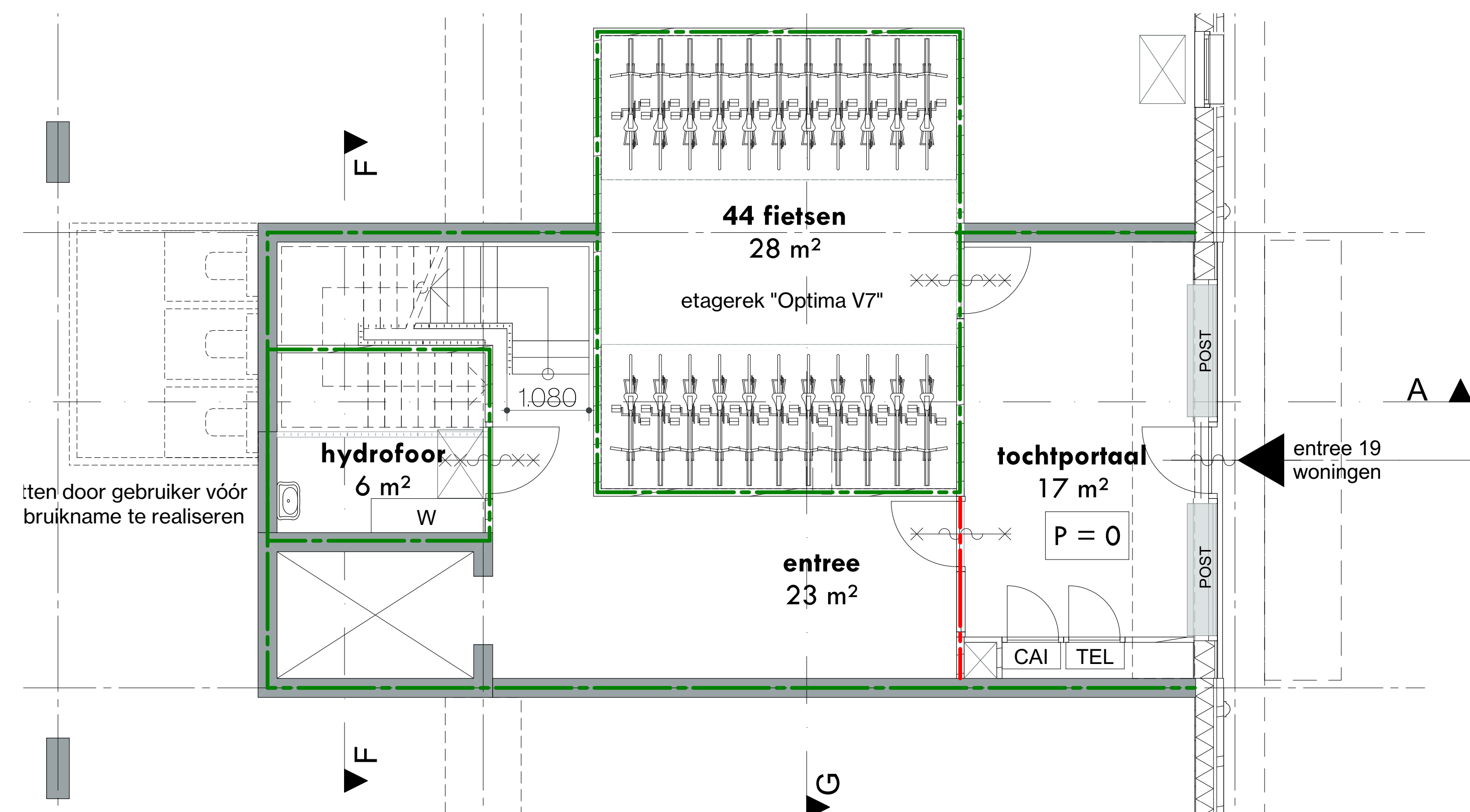
Begane grond
